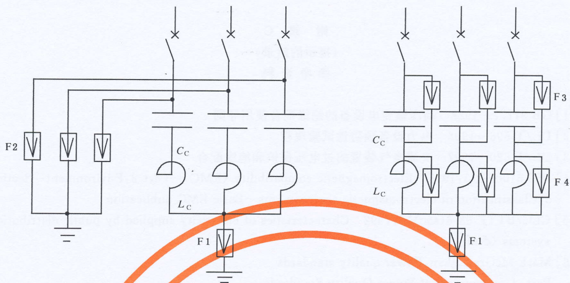
a) 单相重击穿电压的保护接线
