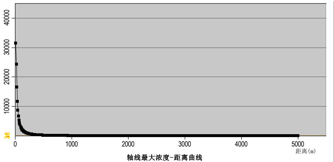
图 7.6-1 泄漏事故下风向不同距离处的最大浓度图（最不利气象条件）
