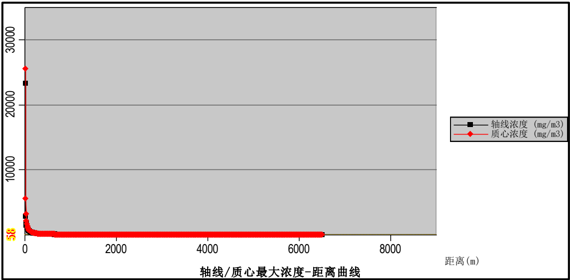
图 7.6-4 泄漏事故下风向不同距离处的最大浓度图（最不利气象条件）
