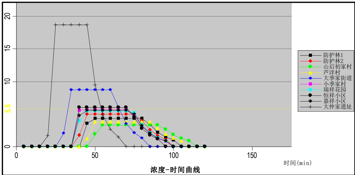
图 7.6-8 在总管接出点泄漏事故各关心点有毒有害物质浓度随时间变化
