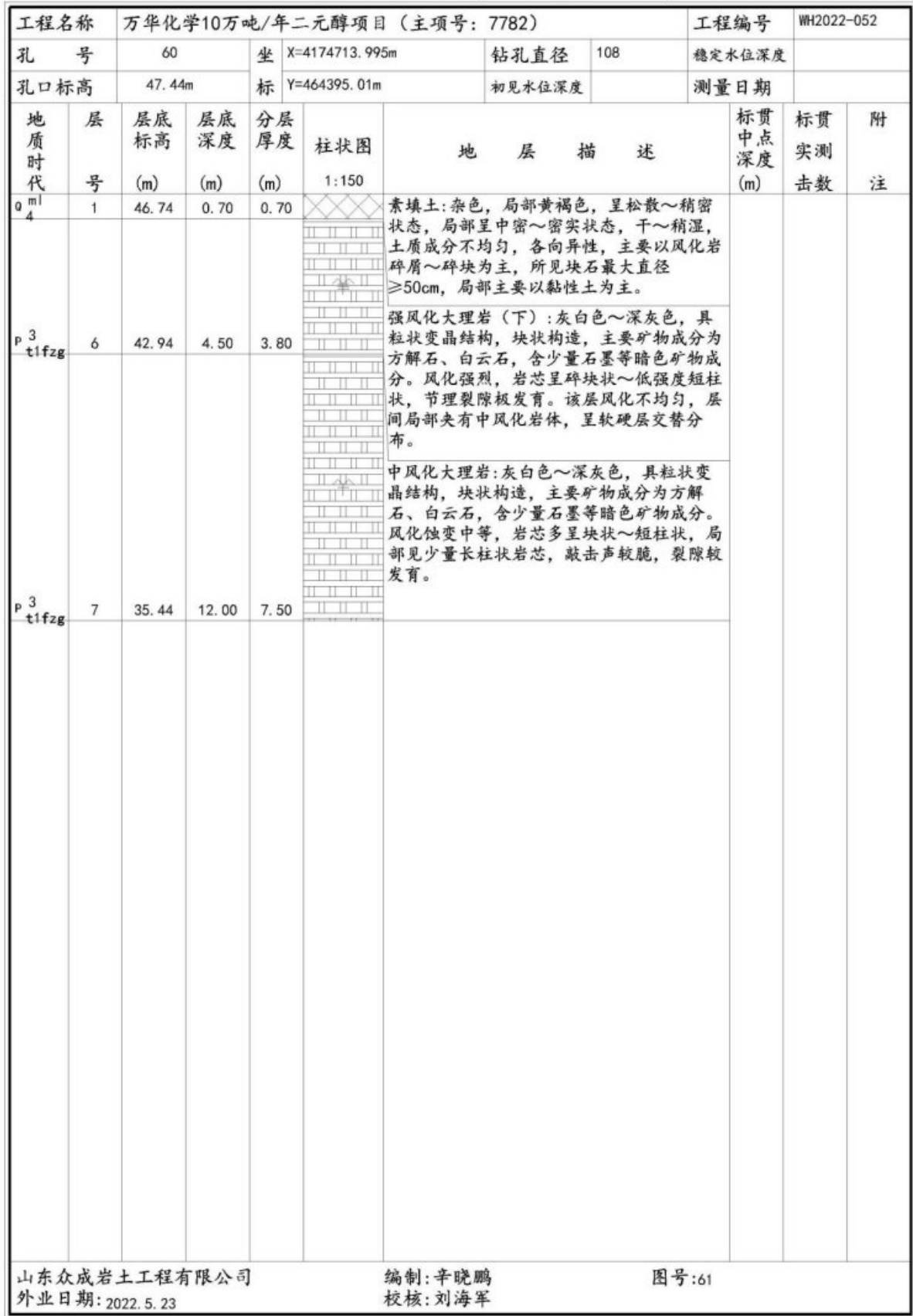
图 6.4-9 60 号井孔结构图
