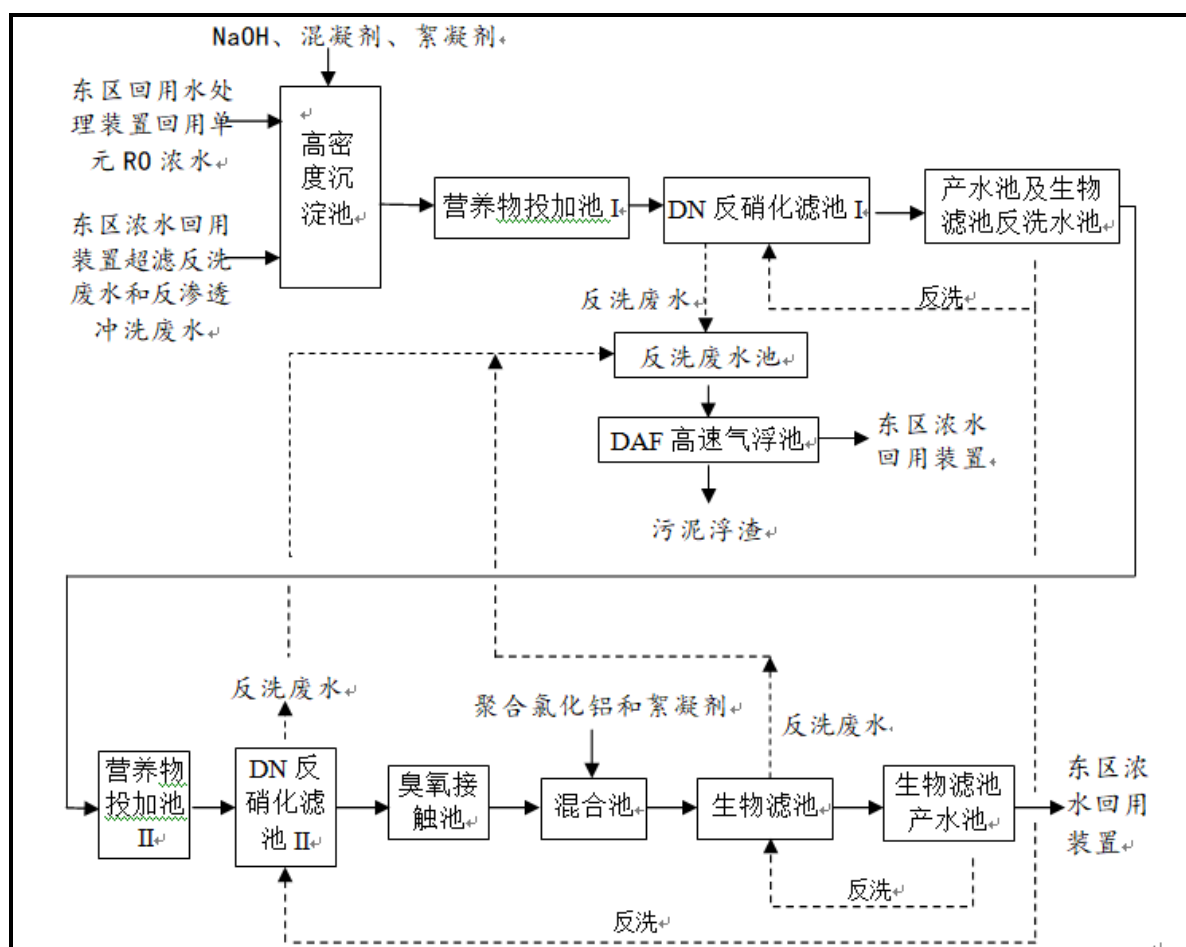
图 4.9-8 东区浓水处理装置工艺流程示意图 (a)
