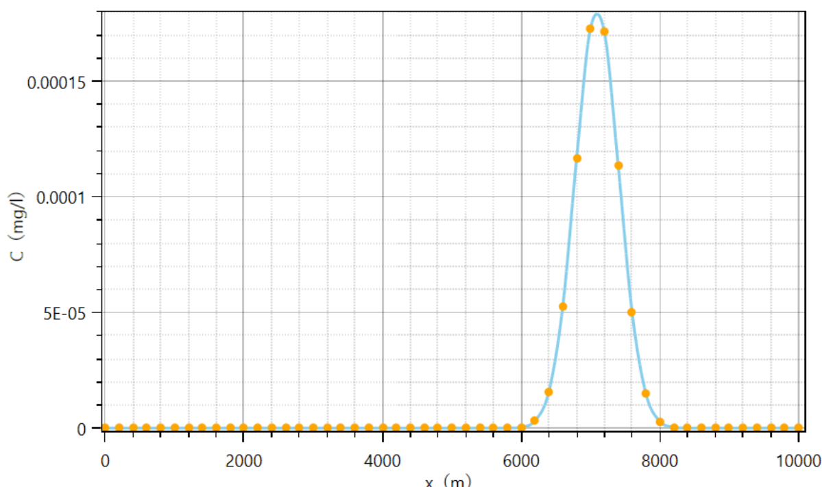
图 6.4-12 7300d 后地下水氟化物浓度和距离关系图
