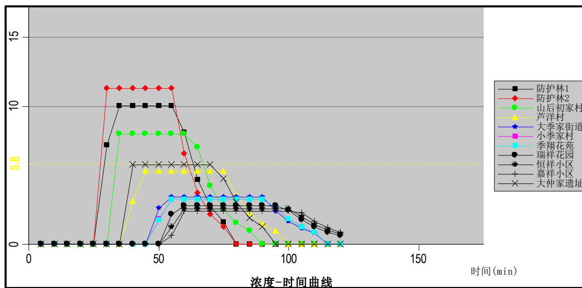
图 7.6-6 装置区泄漏事故各关心点有毒有害物质浓度随时间变化
