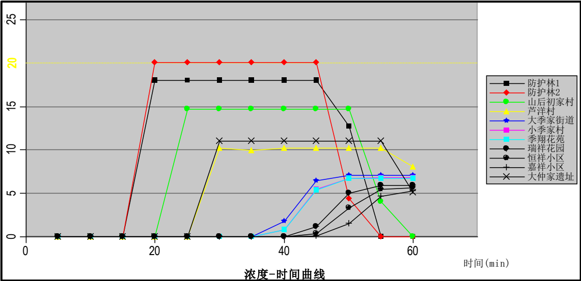
图 7.6-3 泄漏事故各关心点有毒有害物质浓度随时间变化
