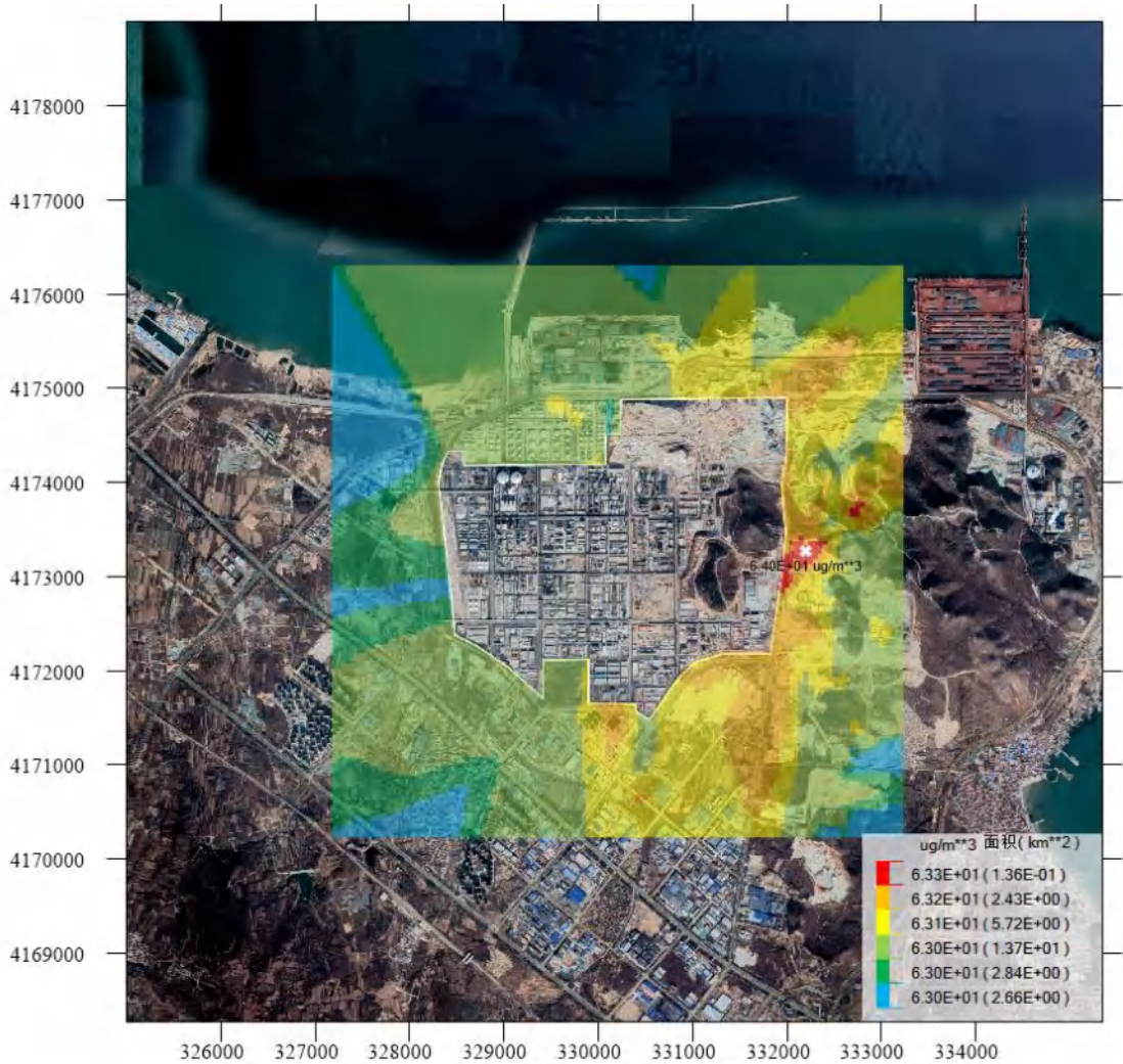
图 5.1-21 叠加后颗粒物（PM 2.5 ）保证率日平均质量浓度分布网格图（ \mu\text{g}/\text{m}^3 ）
