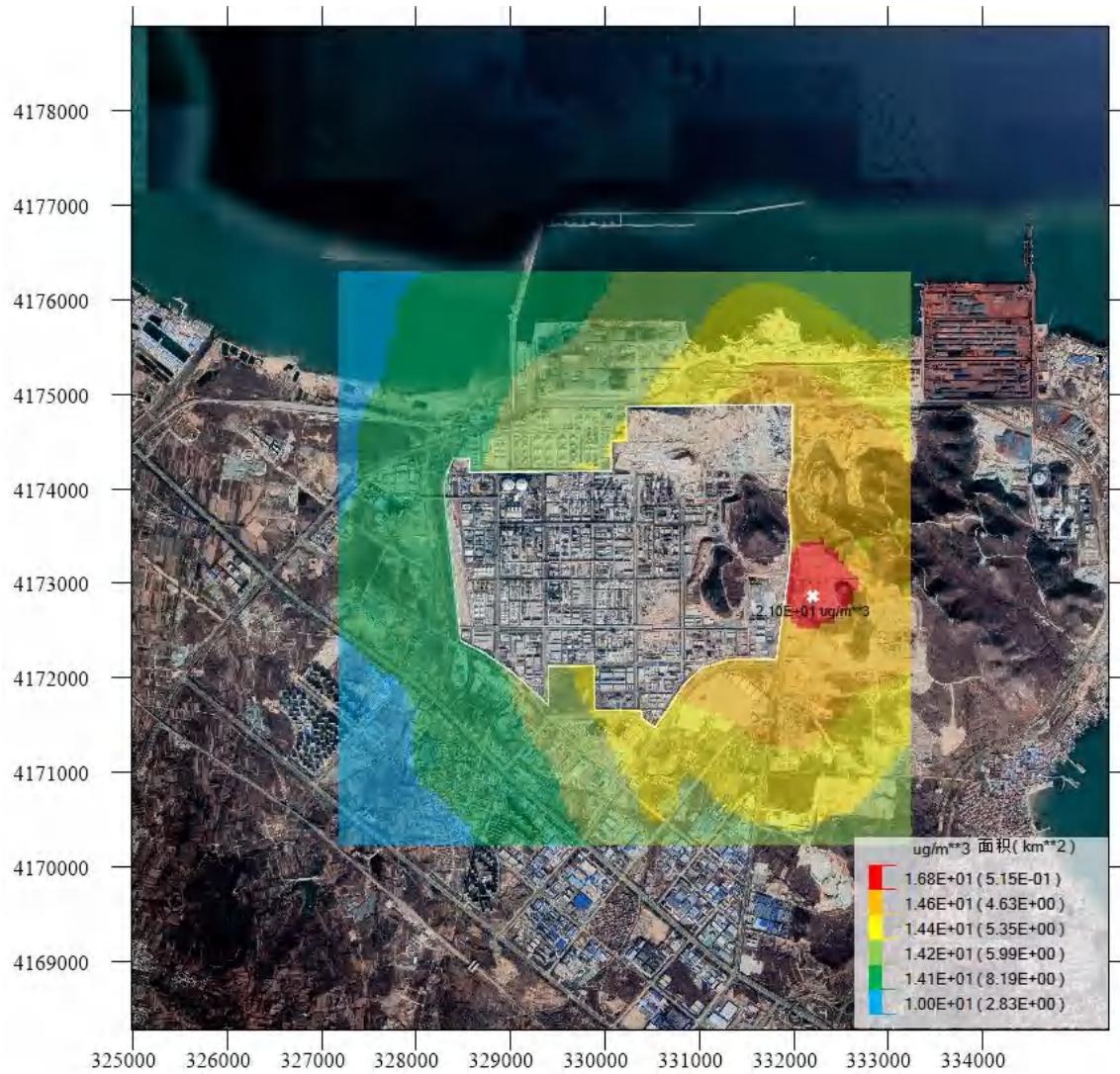
图 5.1-18 叠加后颗粒物（PM 10 ）年平均质量浓度分布网格图（ \mu\text{g}/\text{m}^3 ）
