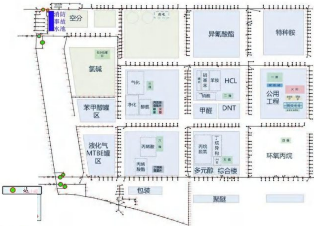
图 6.2-1 现有工程雨排口位置图
