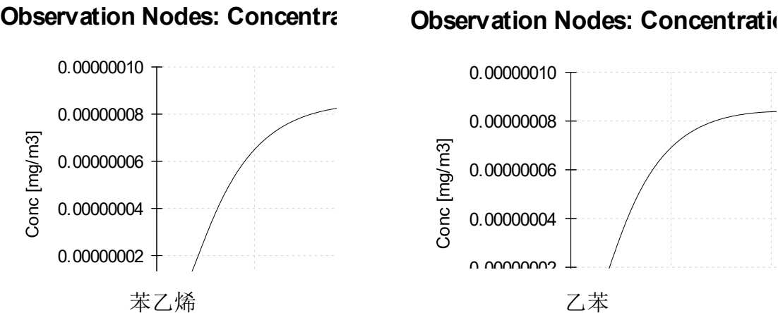
图 5.5-1 非正常工况下土壤不同深度特征污染物浓度随时间变化示意图
