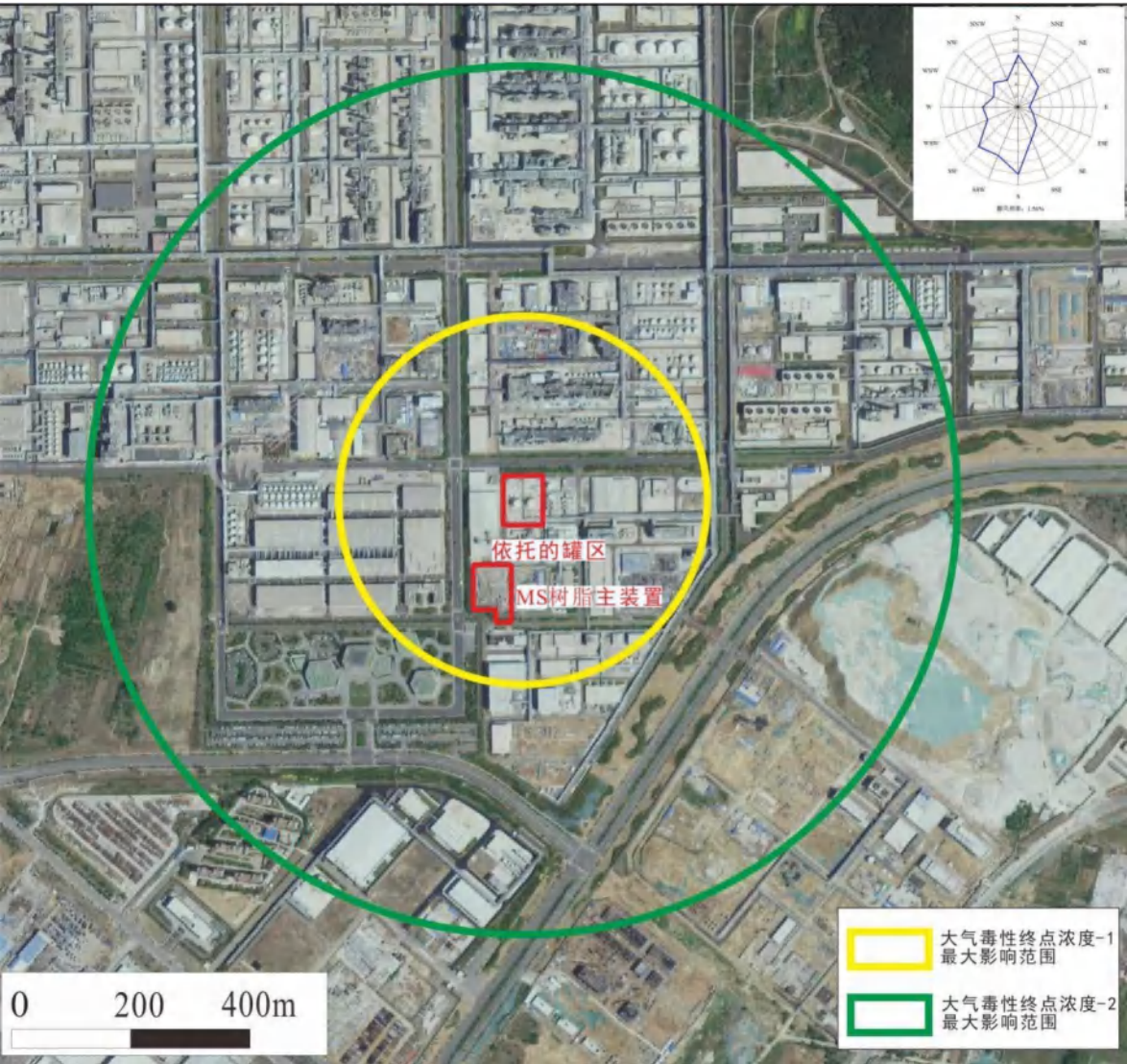
图 6.7-3 发生火灾次生 CO 时最大影响范围图（最不利气象）
