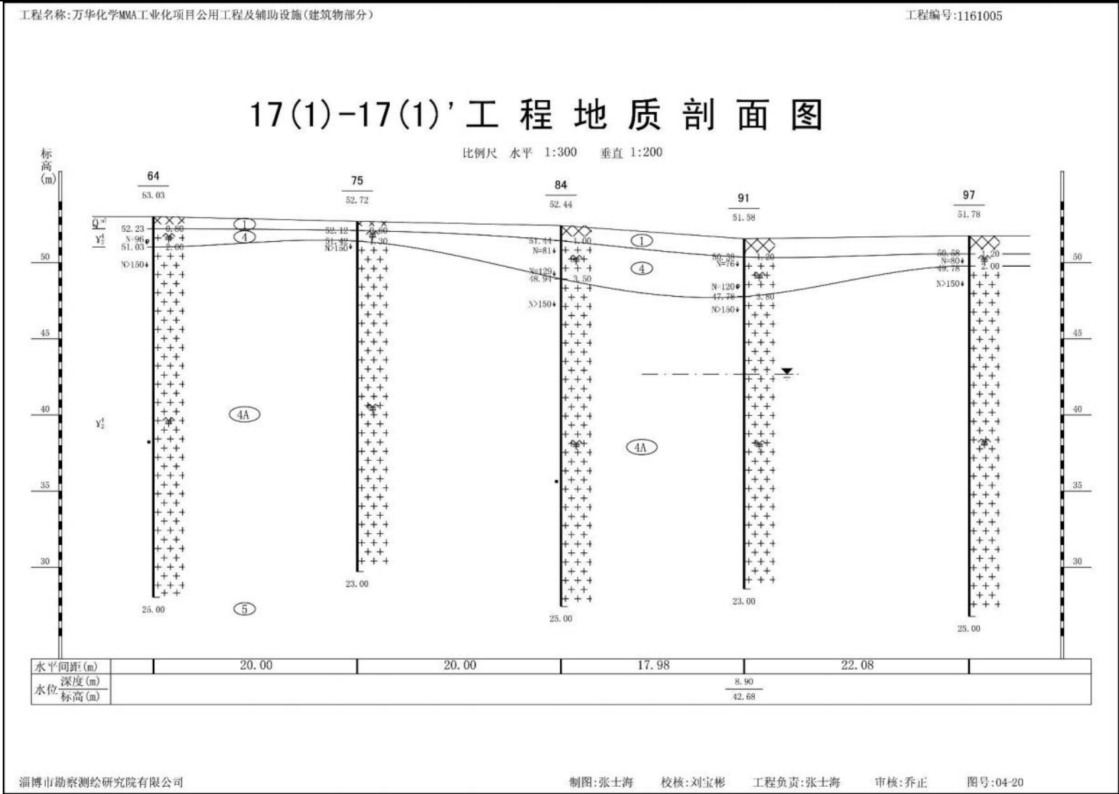
图 5.3-7(3) 17 (1) -17 (1)' 工程地质剖面图
