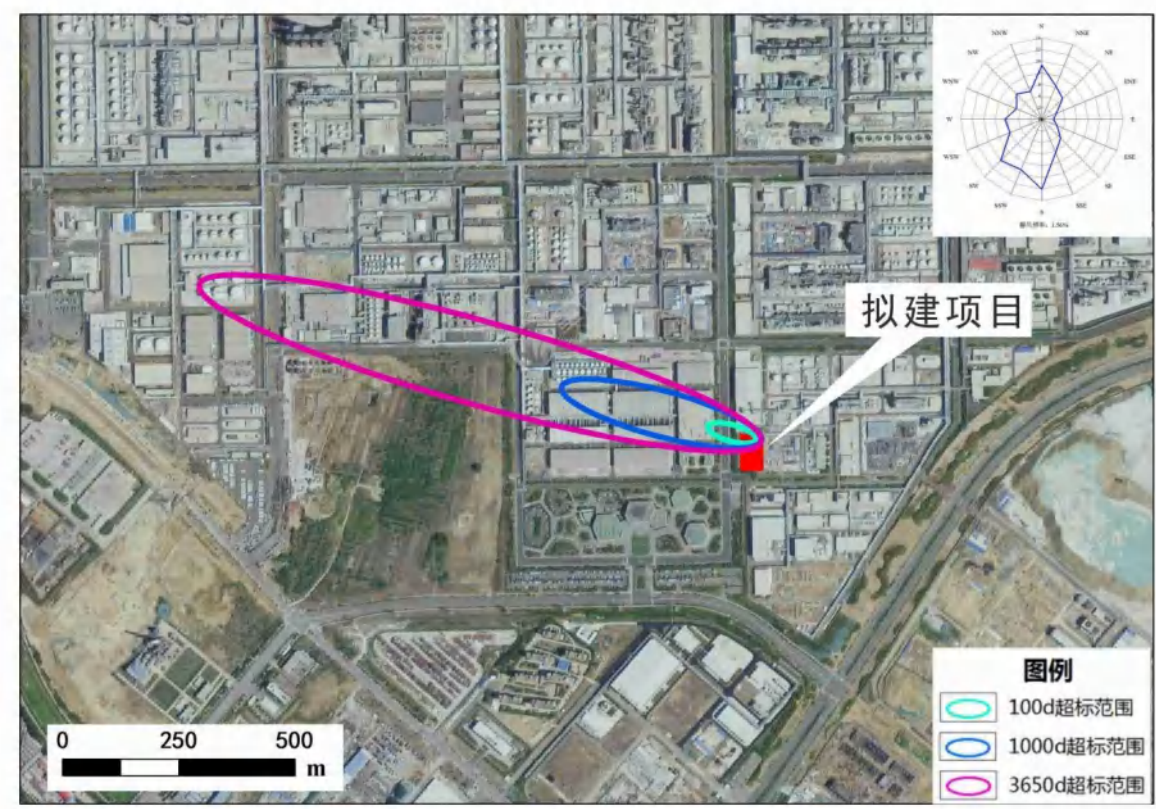
图 5.3-8 工况 1 下 COD Mn 预测结果图
