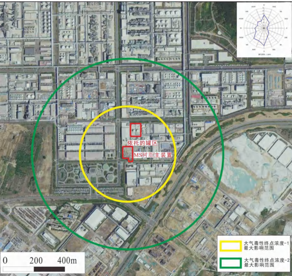
图 6.7-1 MMA 泄漏时最大影响范围图（最不利气象）
