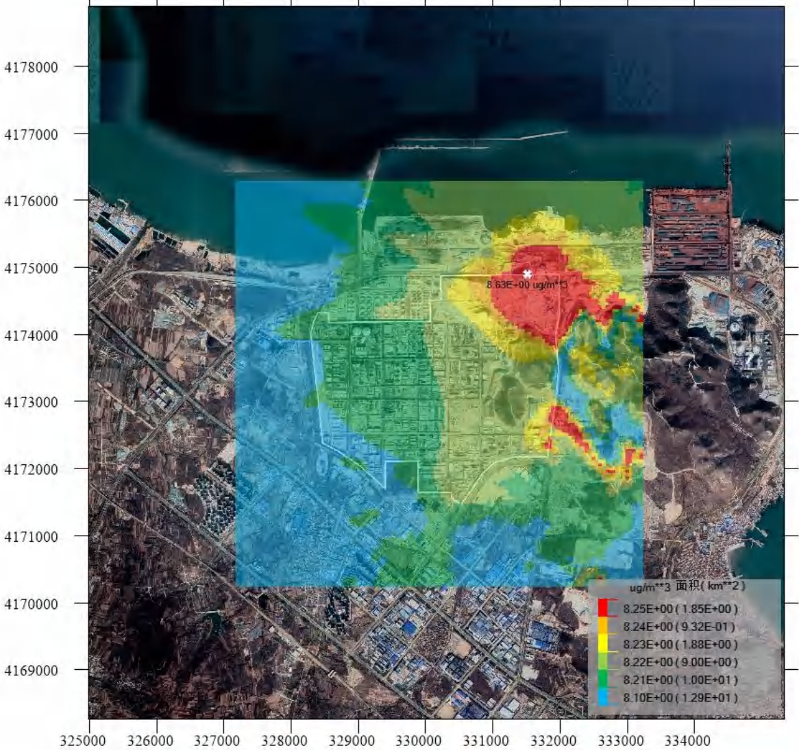
图 5.1-23 叠加后苯乙烯小时平均质量浓度分布网格图 ( \mu\text{g}/\text{m}^3 )
