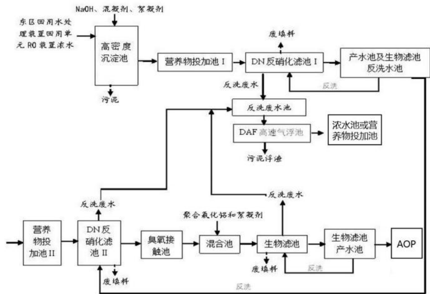
图 2.2-15 东区浓水处理装置工艺流程及产污环节（a）
