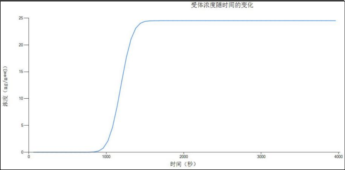
图 6.7-4 发生火灾次生 CO 时大季家村浓度变化图（最不利气象）
