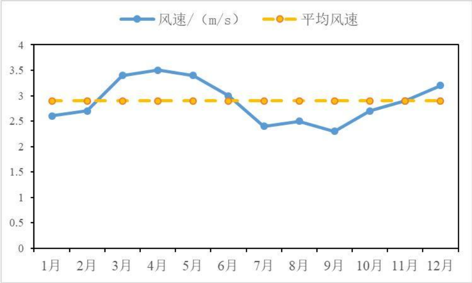
图 5.1-9 2022 年福山站月评价风速的年变化图
