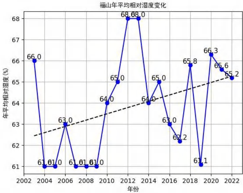
图 5.1-7 福山（2003-2022）年平均相对湿度（纵轴为百分比，虚线为趋势线）
