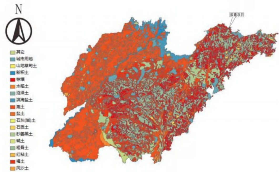
图 4.8-3 山东省土壤类型图
