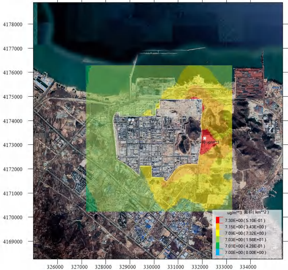
图 5.1-19 叠加后颗粒物（PM 2.5 ）年平均质量浓度分布网格图（ \mu\text{g}/\text{m}^3 ）
