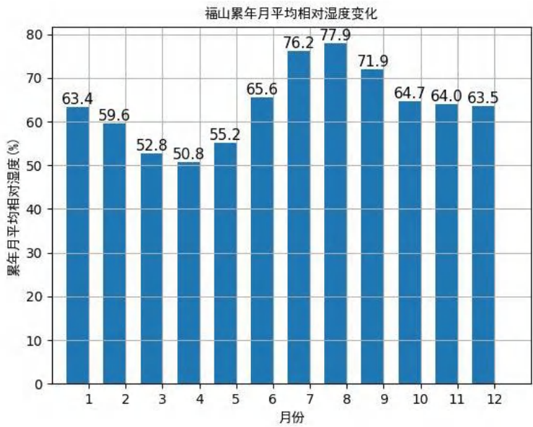
图 5.1-6 福山月平均相对湿度（纵轴为百分比）
