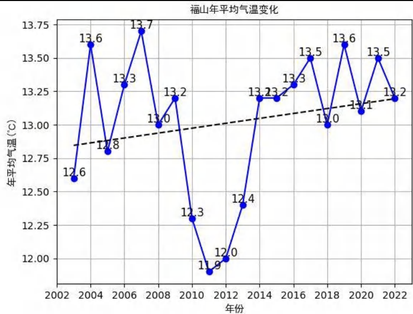
图 5.1-2 福山（2003-2022）年平均气温（单位：℃，虚线为趋势线）
