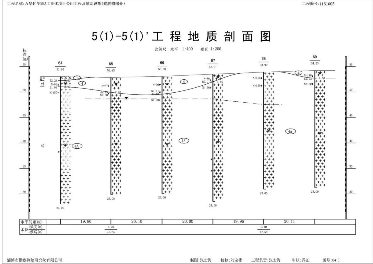
图 5.3-7(2) 5 (1) -5 (1)'工程地质剖面图
