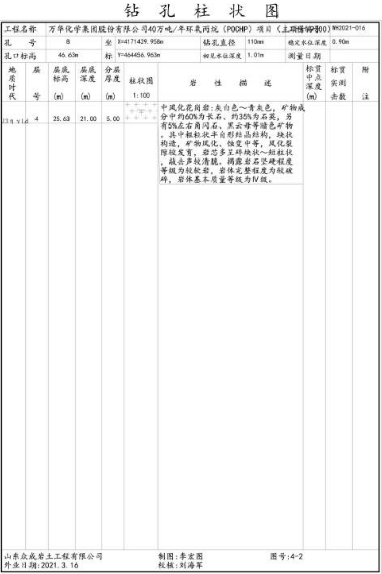
图 6.4-5 钻孔柱状图
