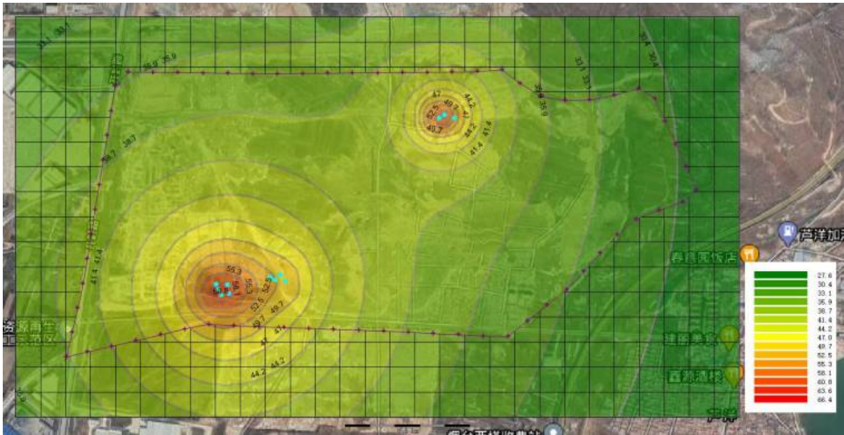
图 6.5-2 本技改项目叠加区域拟建在建噪声贡献值预测结果
