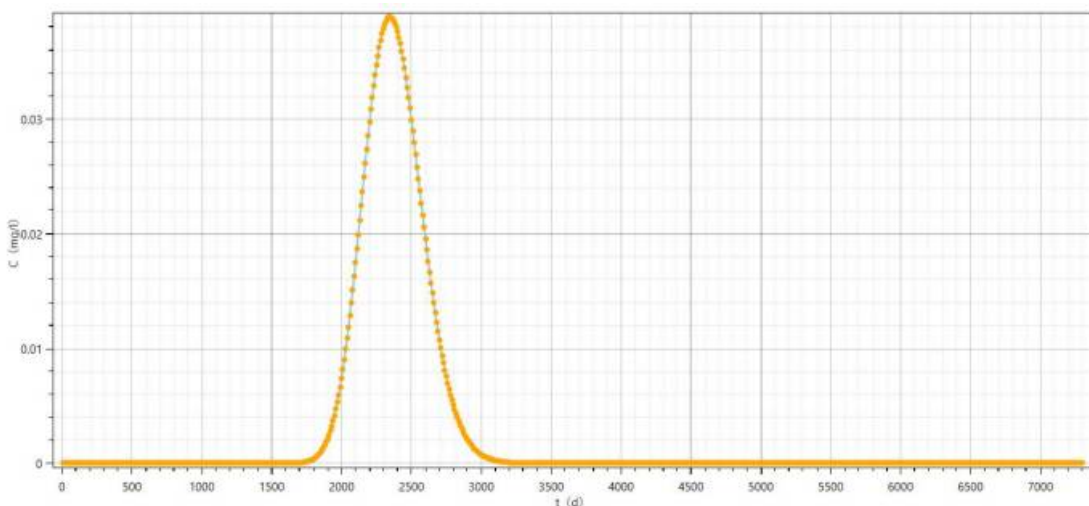
图 6.4-10 西南厂界（地下水流向）处 20 年地下水 COD Mn 浓度和时间关系图
