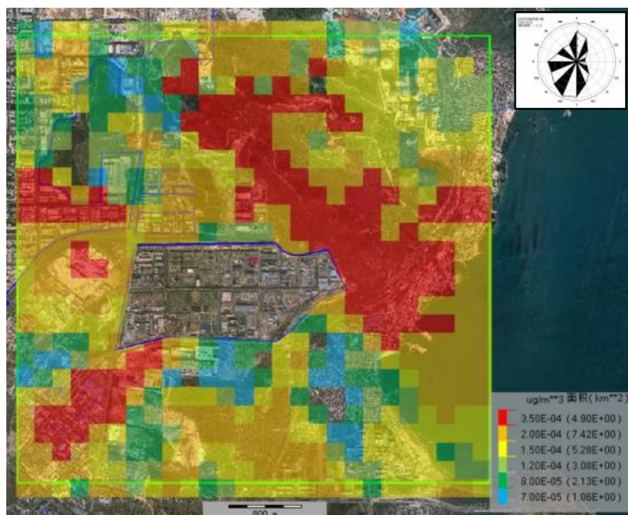
图 6.2-14 CO 日平均贡献质量网格浓度分布图
