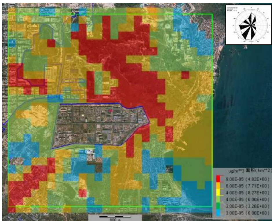
图 6.2-11 PM 2.5 日平均贡献质量网格浓度分布图
