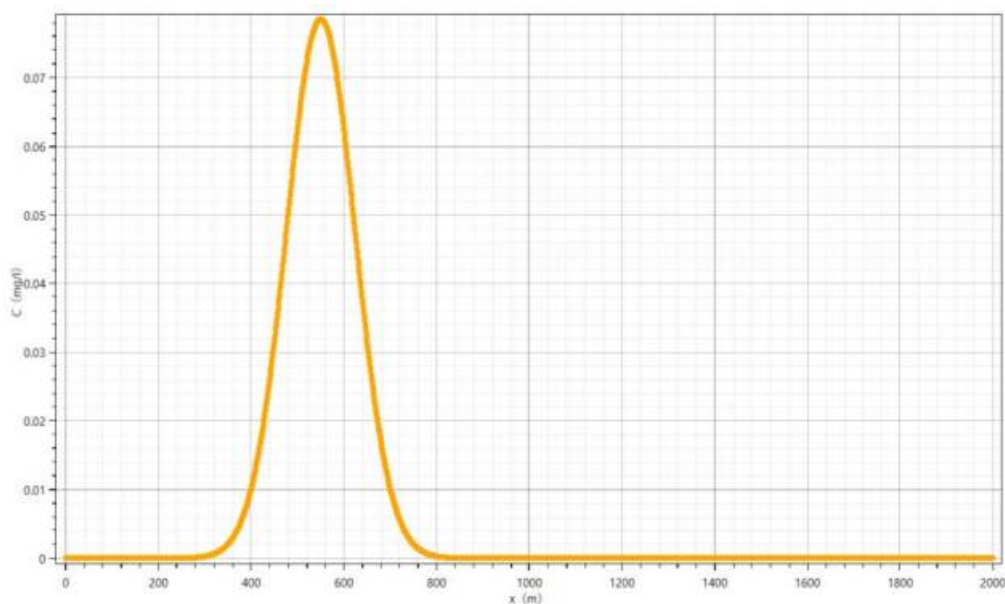
图 6.4-12 废水管线泄漏 1000d 后地下水中 \text{COD}_{\text{Mn}} 浓度和距离关系图
