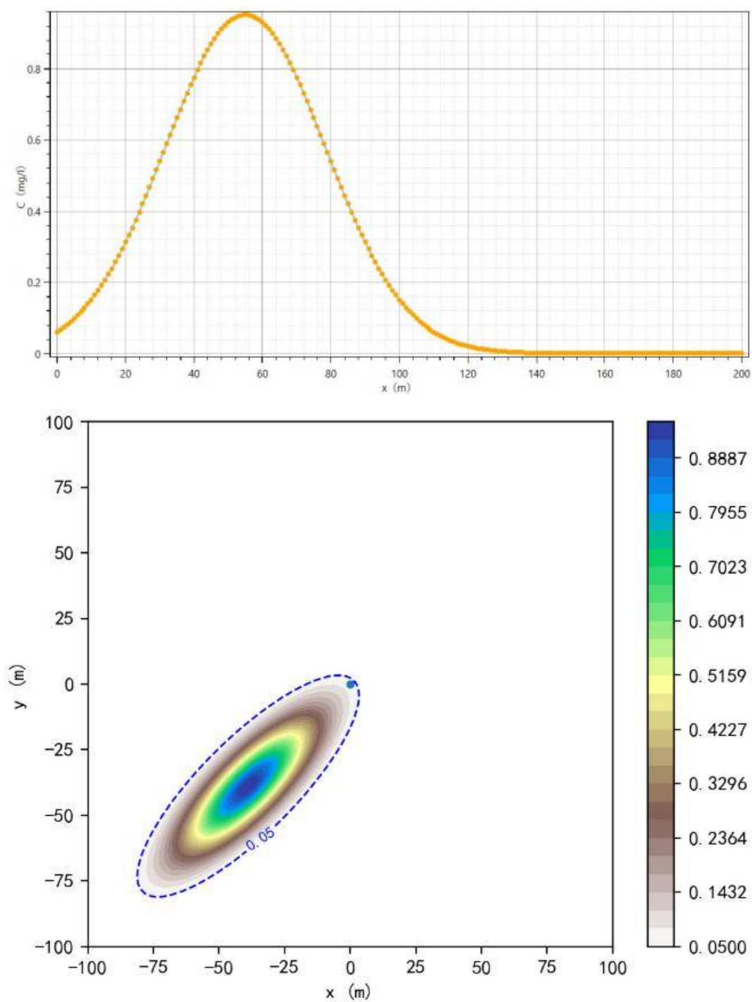
图 6.4-8 废水管线渗漏 100d 后地下水中 \text{COD}_{\text{Mn}} 浓度和距离关系图
