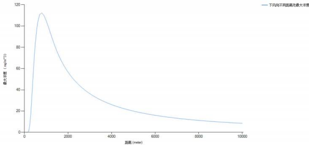
图 7.6-2 MPDO 罐泄漏导致池火事故下风向不同距离处 CO 的最大浓度图（最常见气象）
