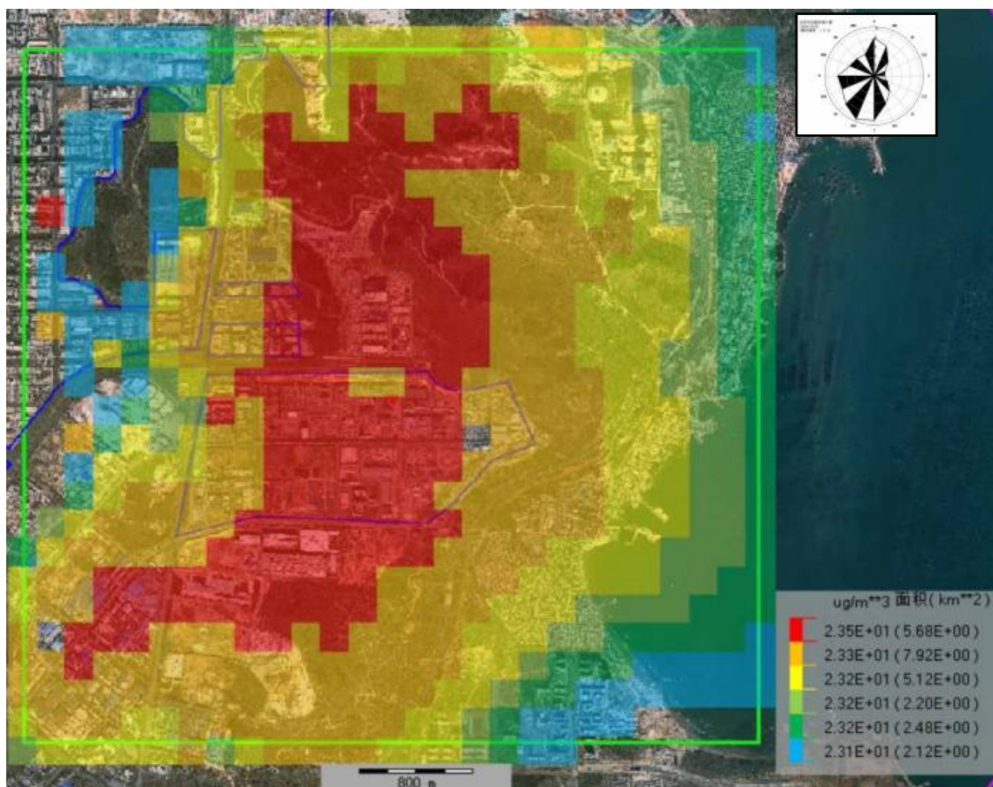
图 6.2-18 叠加后 NO 2 年平均质量网格浓度分布图
