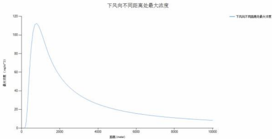
图 7.6-1 MPDO 罐泄漏导致池火事故下风向不同距离处 CO 的最大浓度图（最不利气象）
