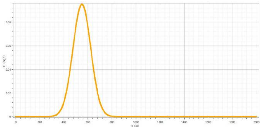
图 6.4-9 废水管线渗漏 1000d 后地下水中 COD Mn 浓度和距离关系图
