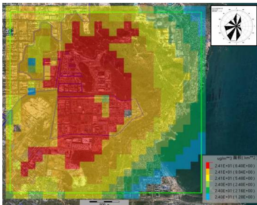
图 6.2-22 叠加后 PM 2.5 年平均质量网格浓度分布图
