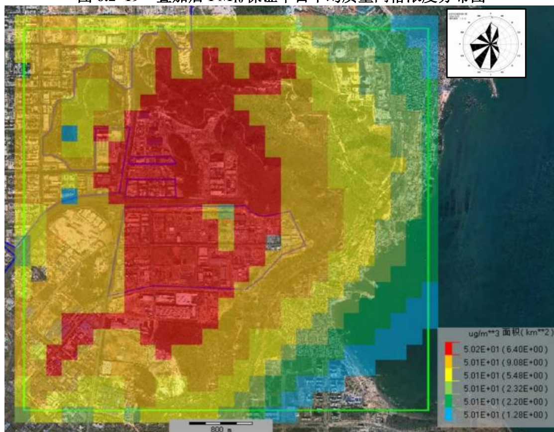
图 6.2-20 叠加后 PM_{10} 年平均质量网格浓度分布图
