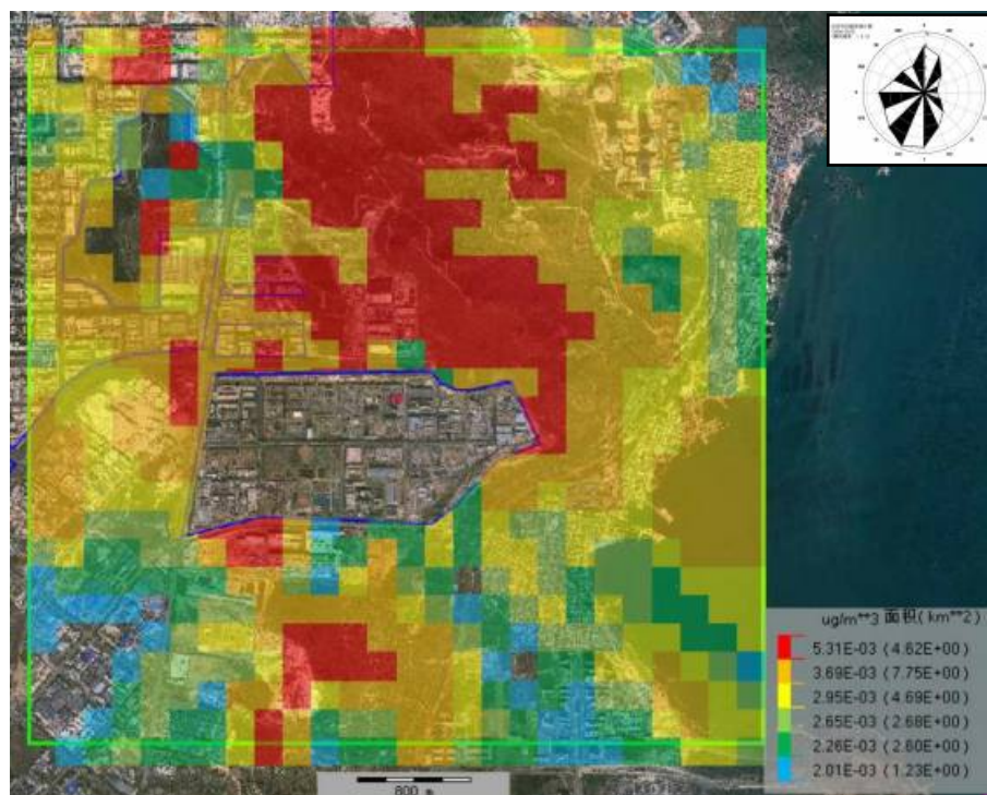
图 6.2-13 CO 小时平均贡献质量网格浓度分布图
