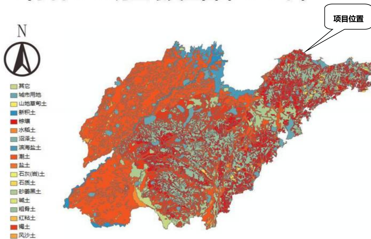
图 5.5-2 土壤类型分布图
