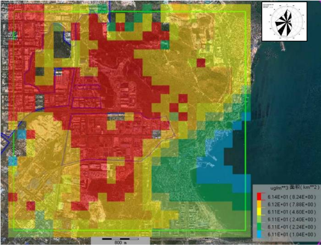
图 6.2-17 叠加后 NO 2 保证率日平均质量网格浓度分布图
