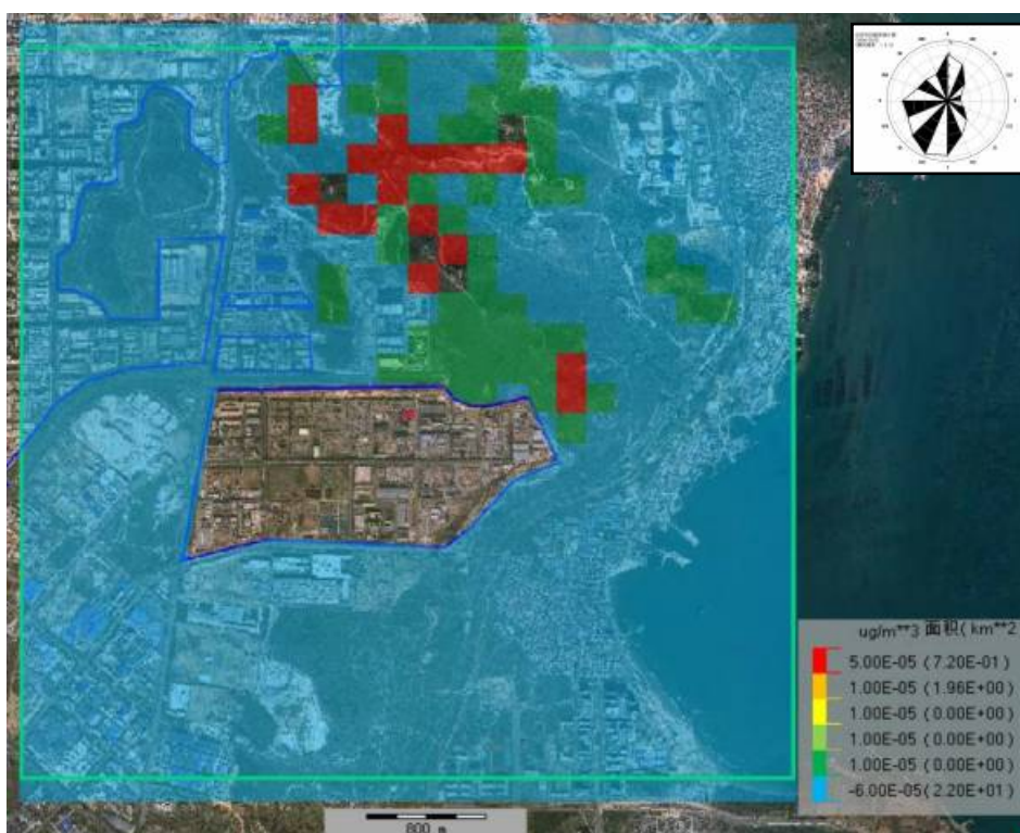
图 6.2-12 PM 2.5 年平均贡献质量网格浓度分布图
