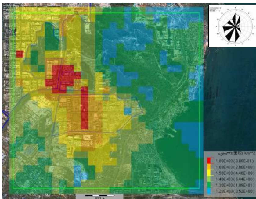
图 6.2-24 叠加后非甲烷总烃小时平均质量网格浓度分布图
