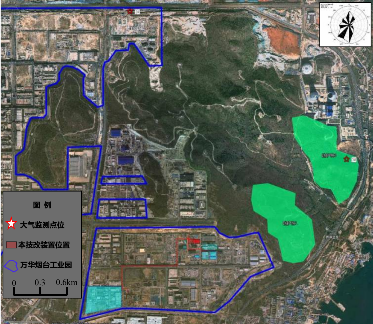
图 5.3-1 环境空气其他污染物监测点位分布图
