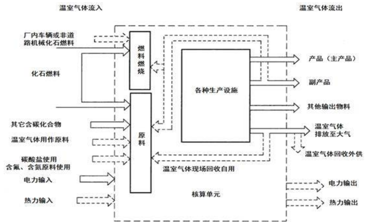
图 4.11-1 化工行业温室气体源流识别示意图
