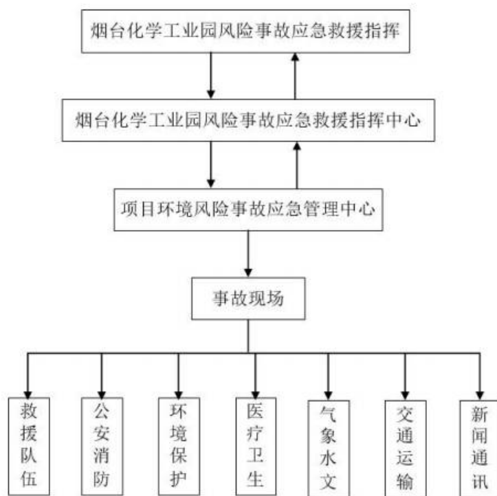
图 7.7-4 烟台化工产业园突发环境事件应急预案体系图
