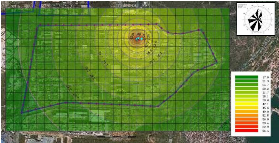
图 6.5-1 本技改项目噪声贡献值预测结果
