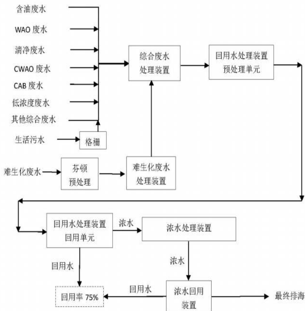
图 3.2-8 万华环保科技东区污水处理站处理单元设置示意图
