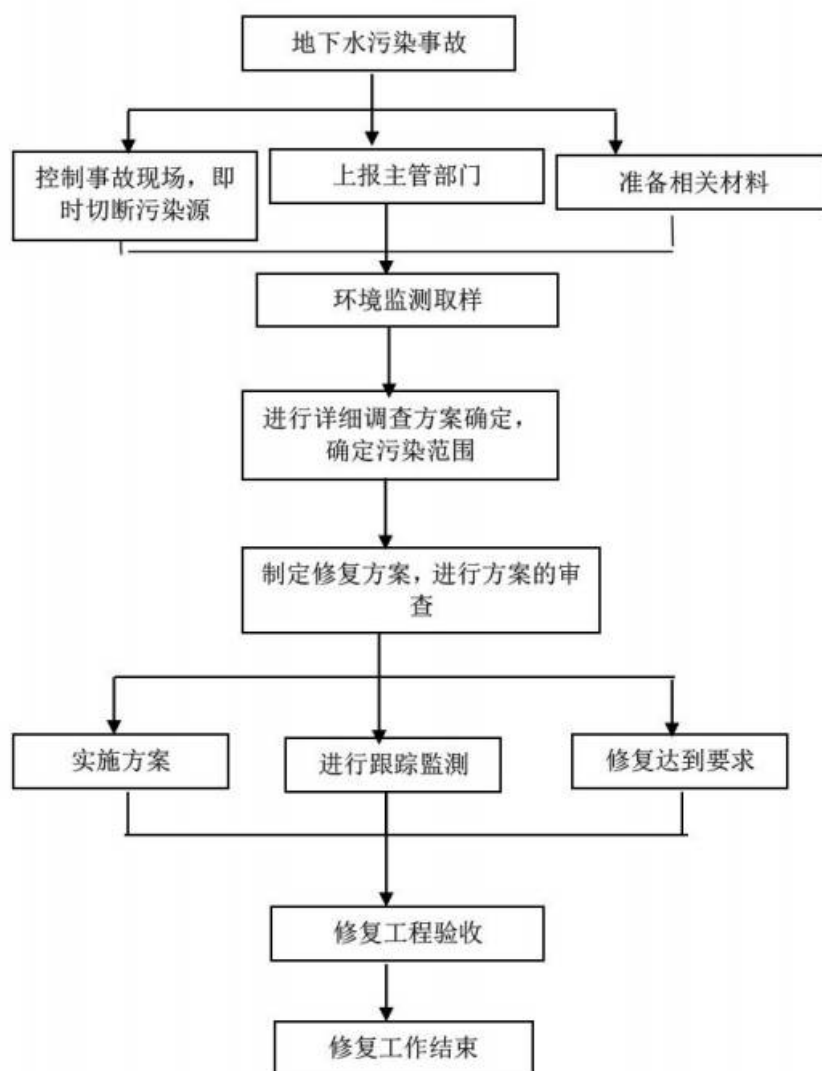
图 8.2-13 地下水污染应急响应程序框图
