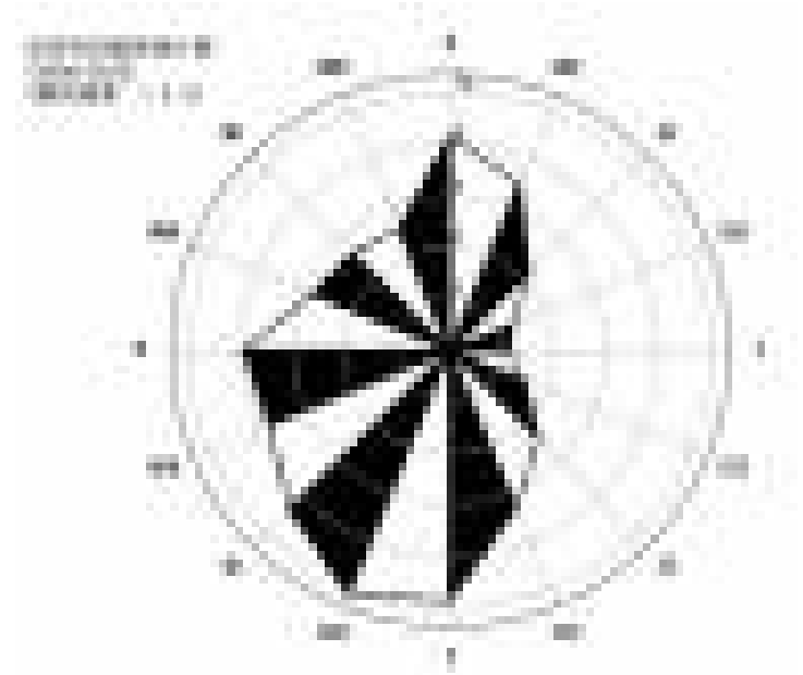
图 6.2-2 福山站近 20 年（2004-2023 年）风向玫瑰图（静风频率 1.0%）
