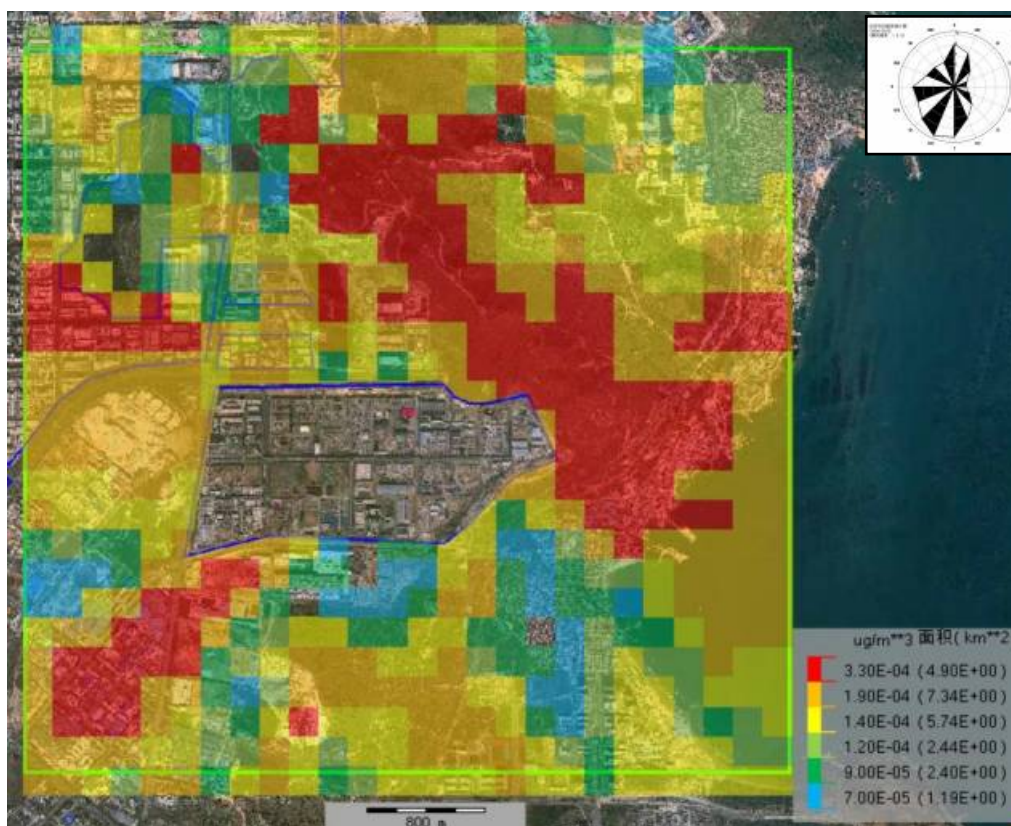
图 6.2-7 \text{NO}_2 日平均贡献质量网格浓度分布图
