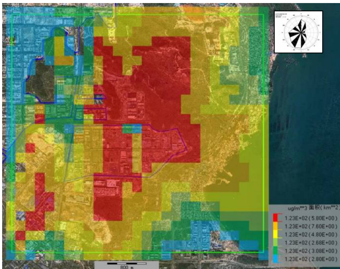
图 6.2-19 叠加后 PM_{10} 保证率日平均质量网格浓度分布图
