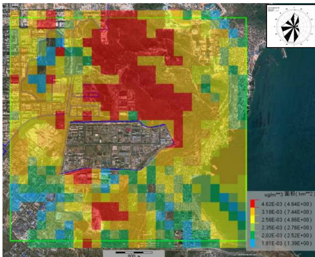
图 6.2-6 \text{NO}_2 小时平均贡献质量网格浓度分布图
