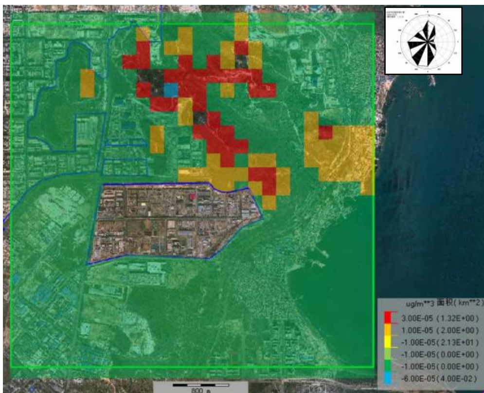
图 6.2-10 PM_{10} 年平均贡献质量网格浓度分布图
