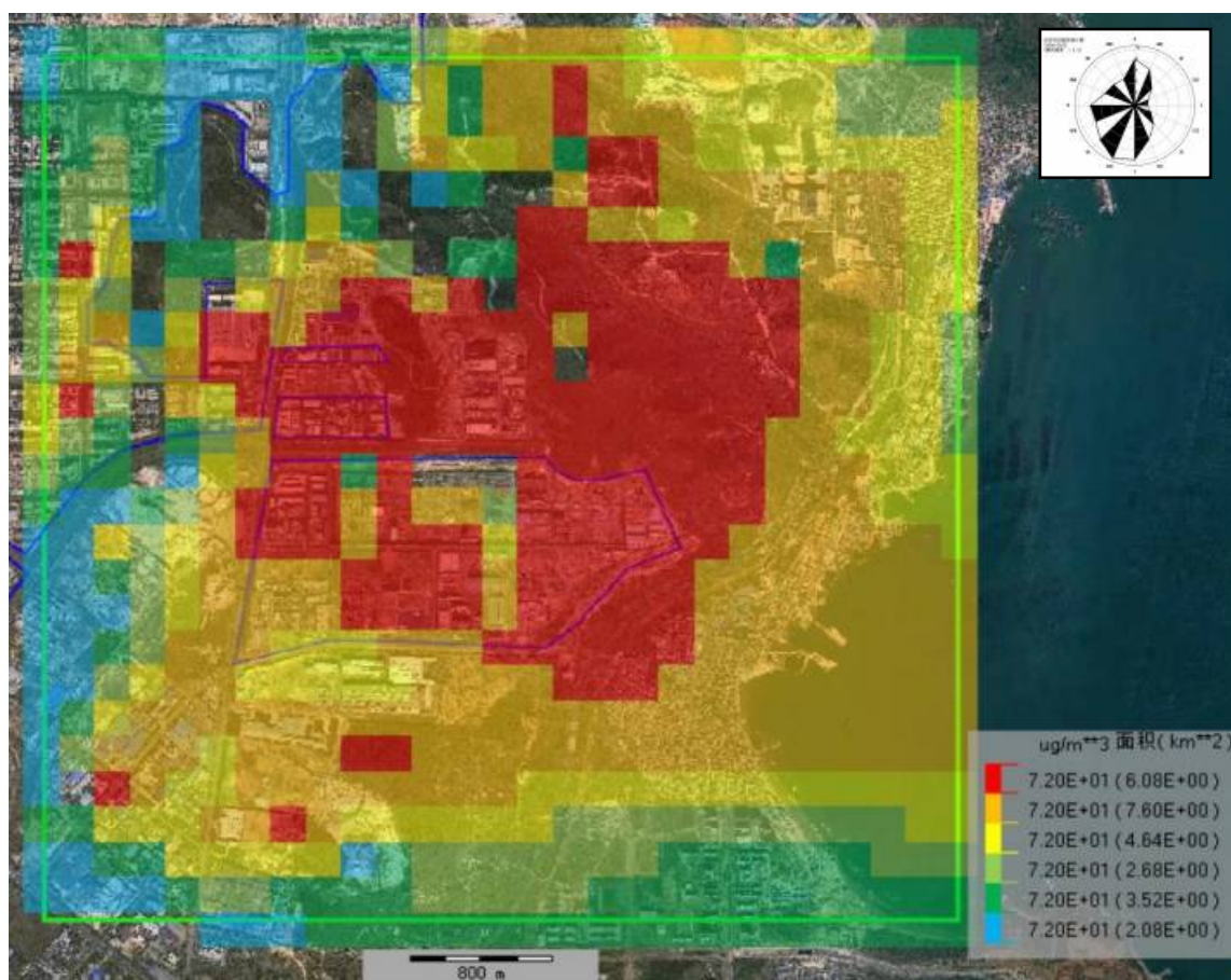
图 6.2-21 叠加后 PM 2.5 保证率日平均质量网格浓度分布图
