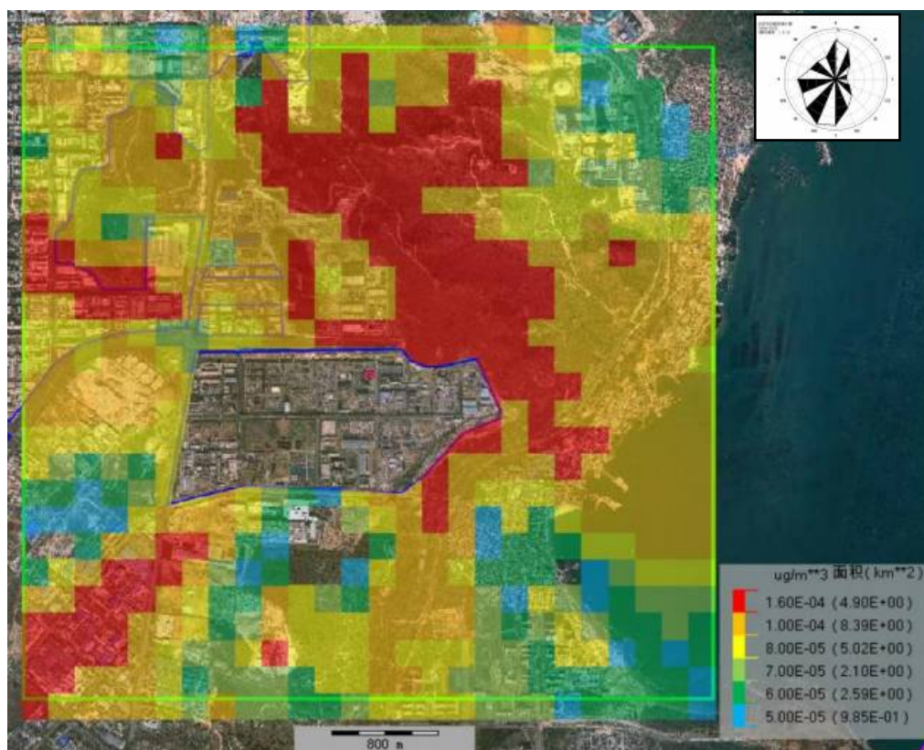
图 6.2-9 \text{PM}_{10} 日平均最大贡献质量网格浓度分布图
