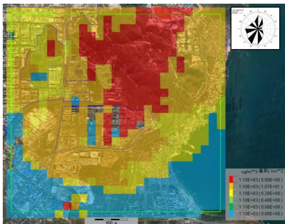
图 6.2-23 叠加后 CO 保证率日平均质量网格浓度分布图
