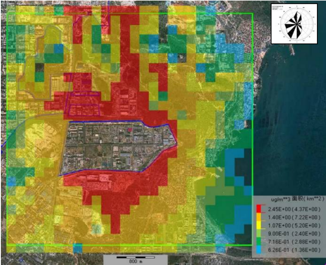
图 6.2-15 非甲烷总烃小时平均质量浓度分布图
