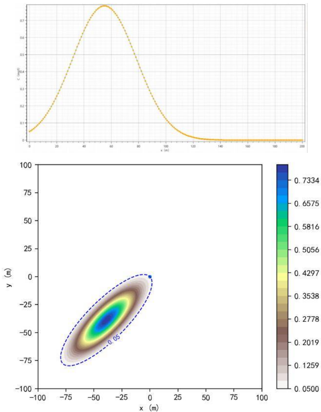
图 6.4-11 废水管线泄漏 100d 后地下水中 \text{COD}_{\text{Mn}} 浓度和距离关系图
