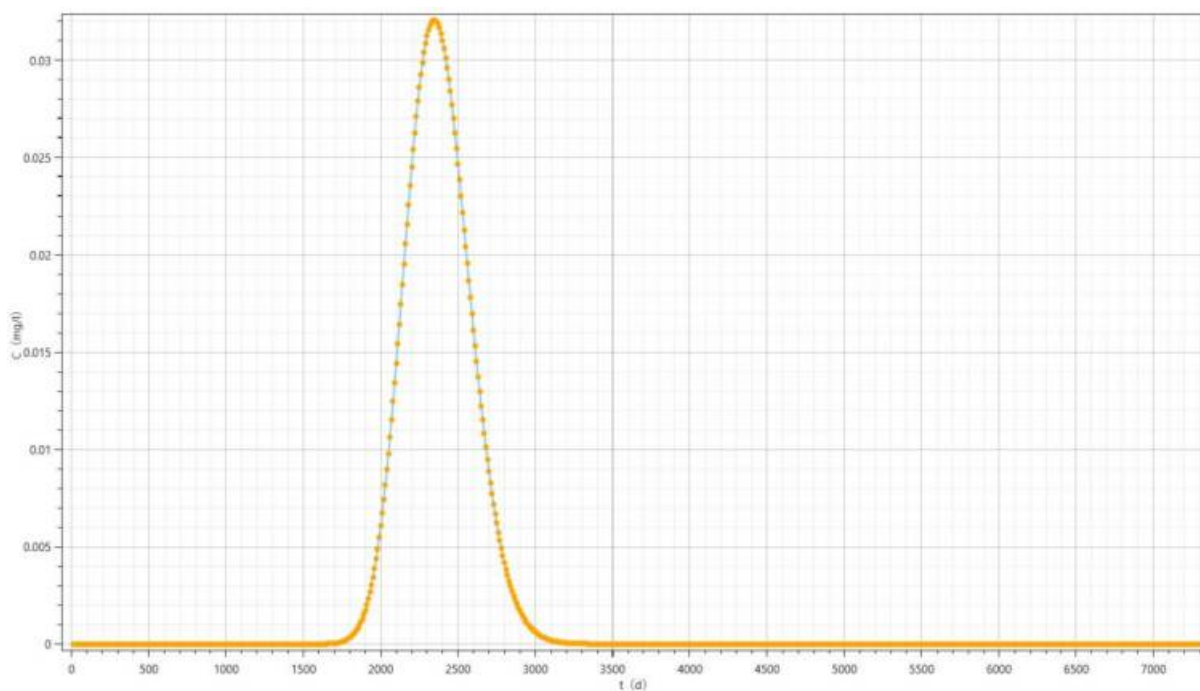
图 6.4-13 西南厂界（地下水流向）处 20 年地下水中 \text{COD}_{\text{Mn}} 浓度和时间关系图
