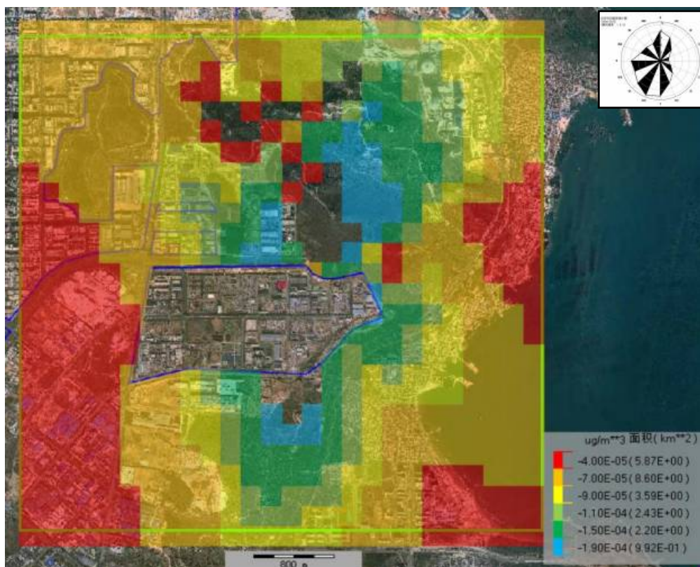
图 6.2-8 \text{NO}_2 年平均贡献质量网格浓度分布图
